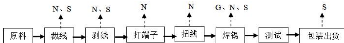
图 3-3 项目生产工艺及产污环节流程图
